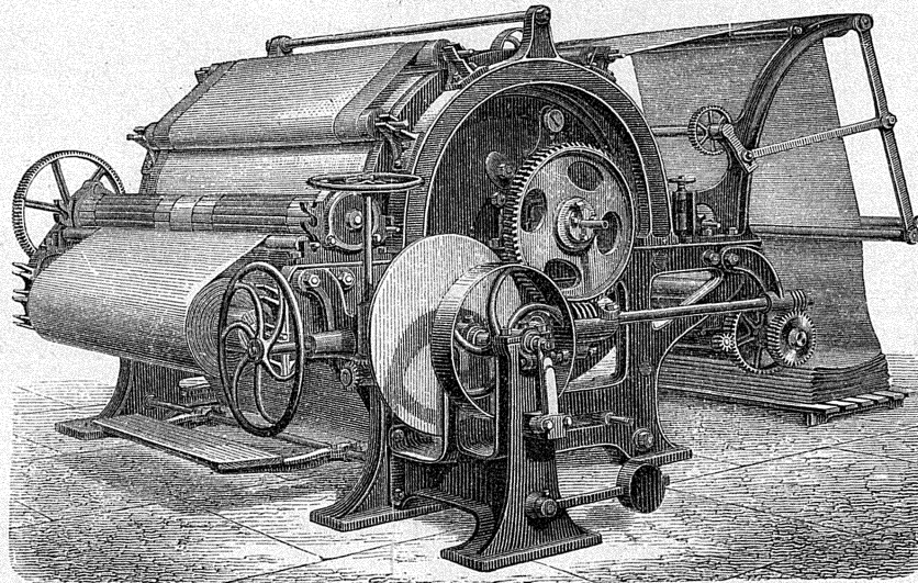
6. Паровая сушильная машина.
