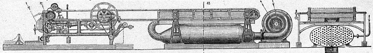
5. Рамочная (отажная) сушилка.
