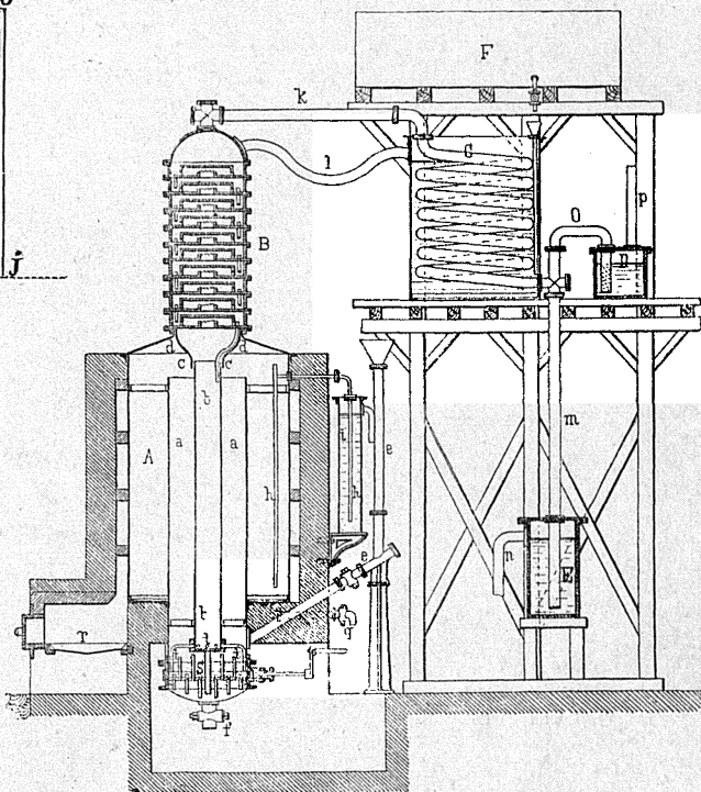
Аппаратъ для дестилляціи (Къ ст. Аммоніумъ).
