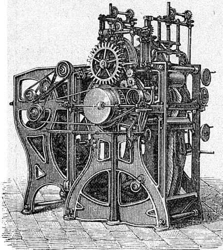
3. Универсальная валавая машина.
